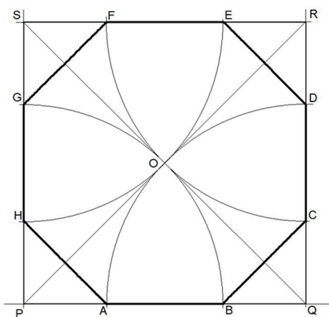
Octàgon inscrit en un quadrat
